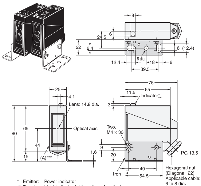
E3JM-10□4T
