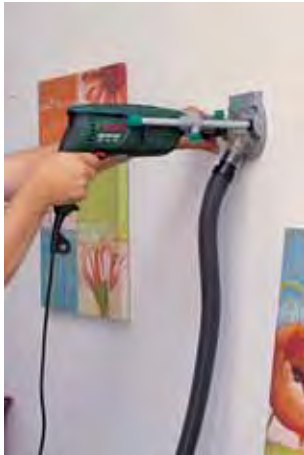
mit Anschluß für Staubabsaugung - in jeder Lage staubfrei und präzise Bohren
