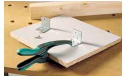
große Spanntiefe erlaubt auch Fixieren in randfernen Bereichen
